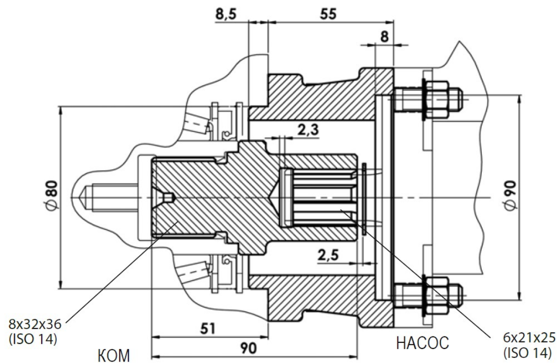
Адаптер-переходник KOM ISO на насос НШ
